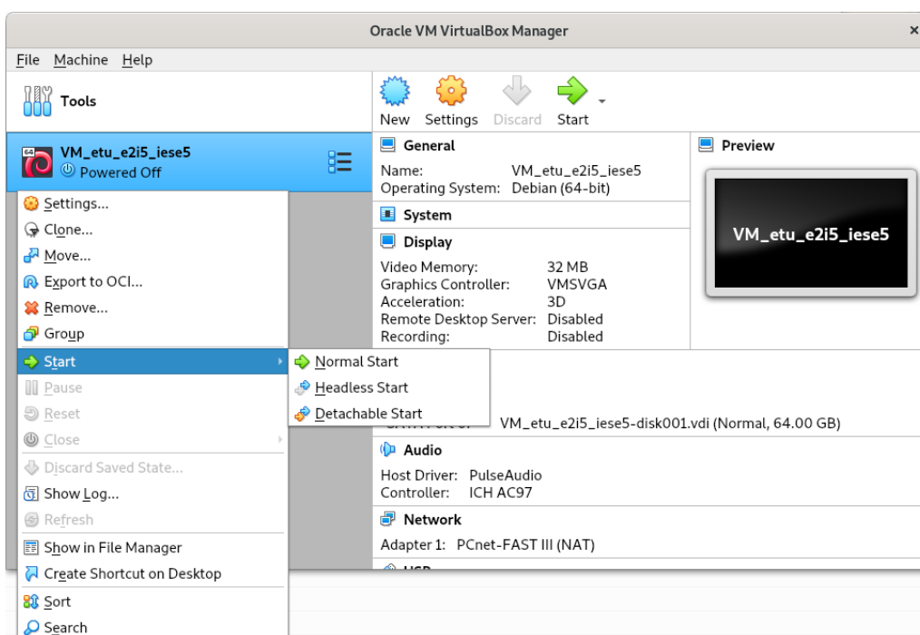
FIGURE 5 – Démarrer la VM étudiant IESE5
